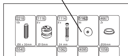
Beschlagteile/fitings
